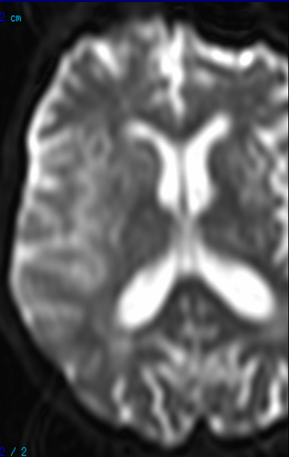
EPI-SE-T2
