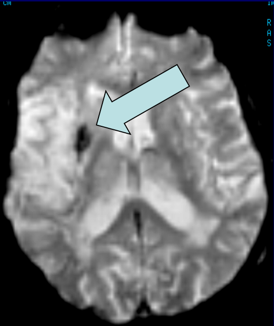
EPI-GRE-T2*
