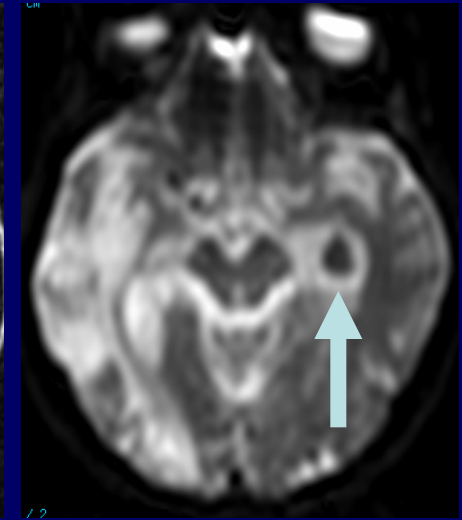
EPI-SE-T2
