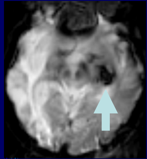
EPI-GRE-T2*
